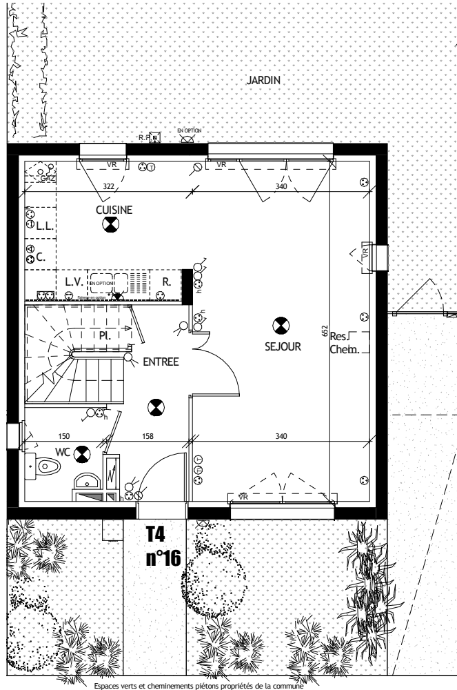
REZ-DE-CHAUSSEE
